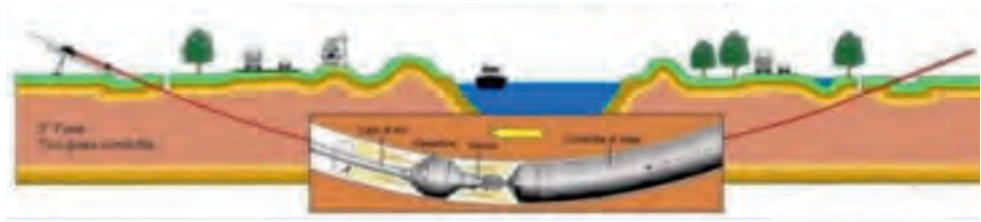
TRIVELLAZIONE ORIZZONTALE CONTROLLATA
