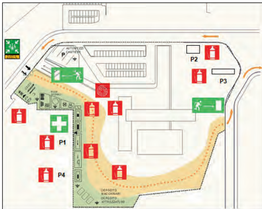
PLANIMETRIA DELL'ORGANIZZAZIONE DEL CANTIERE AI FINI ANTINCENDIO
